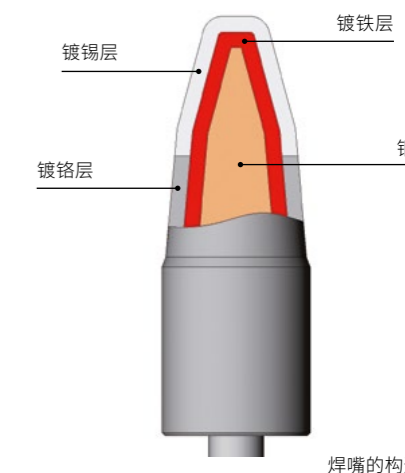
焊嘴的构造
