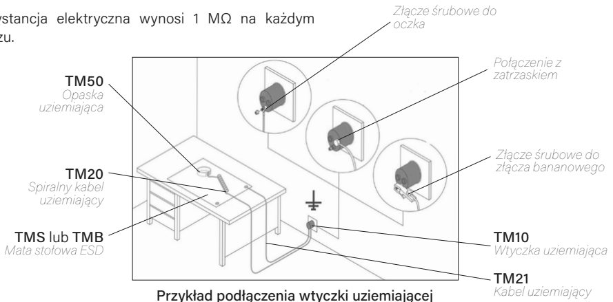
Przykład podłączenia wtyczki uziemiającej
