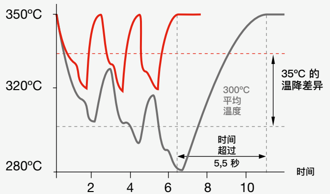
高效的温度控制 3 种焊点的对比工艺
