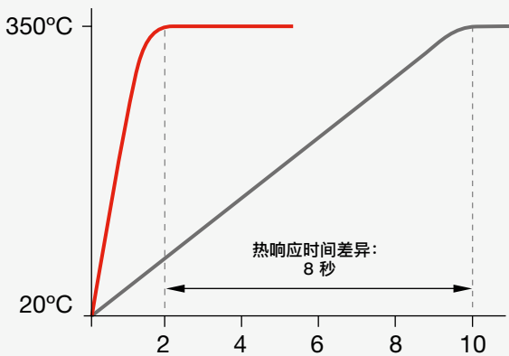
2 秒内达到 350°C
