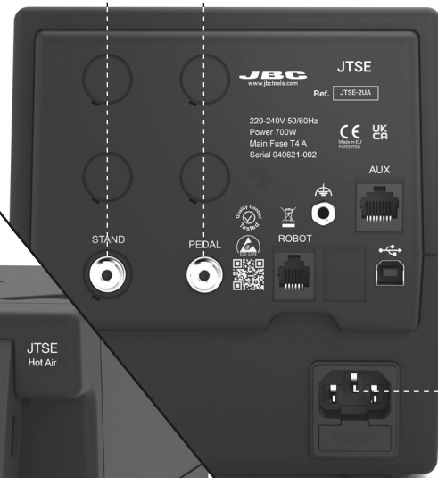
后视图
