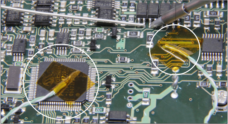
Hilfthermoelement (TC)
